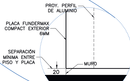
DETALLE 3 SEPARACIÓN AL PISO SIN ESCALA
