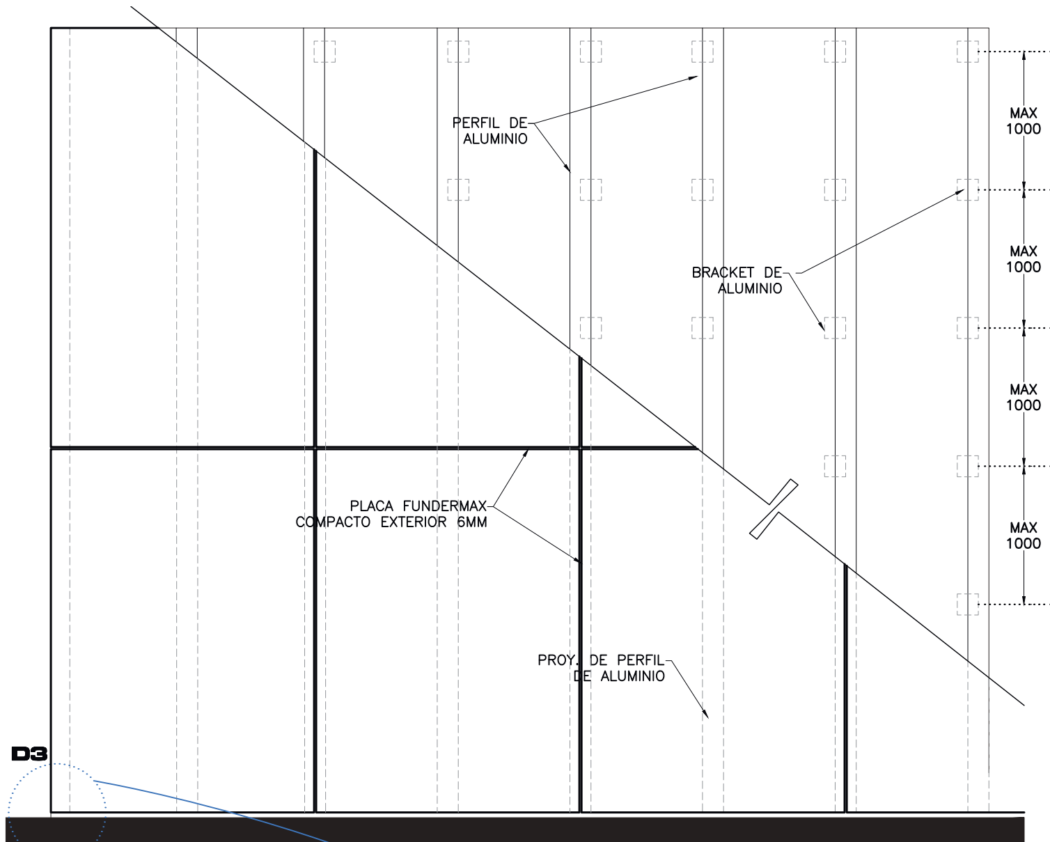
DETALLE 3 SEPARACIÓN AL PISO SIN ESCALA
